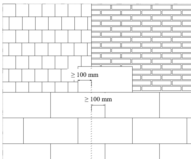
3 paveikslas. Termoizoliacinių gaminių klėjavimas dviejų skirtingų pagrindo medžiagų sandūroje
