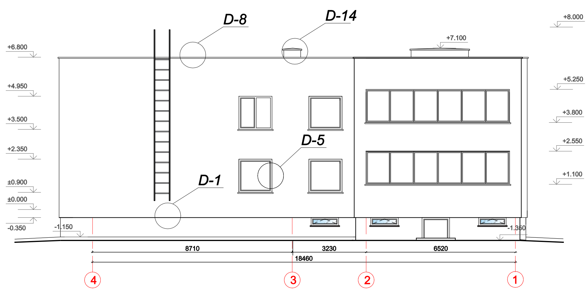
FASADAS TARP AŠIŲ "4-1" M 1:100
