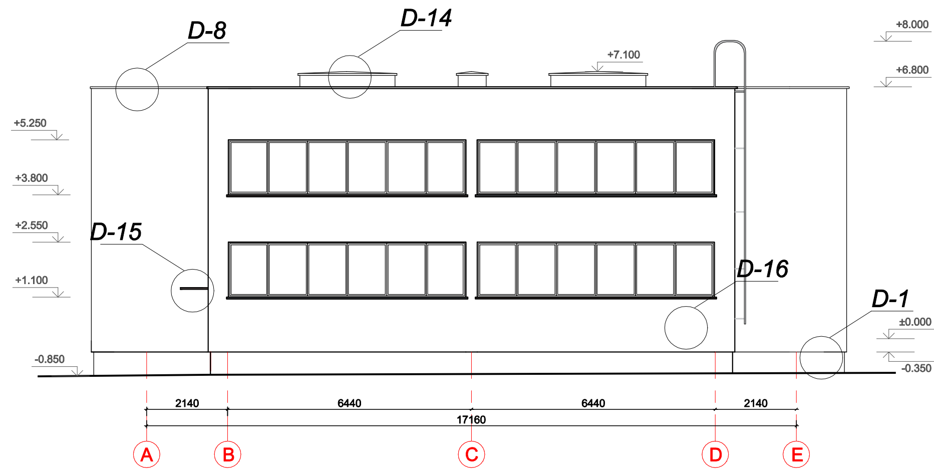
FASADAS TARP AŠIŲ "A-E" M 1:100
