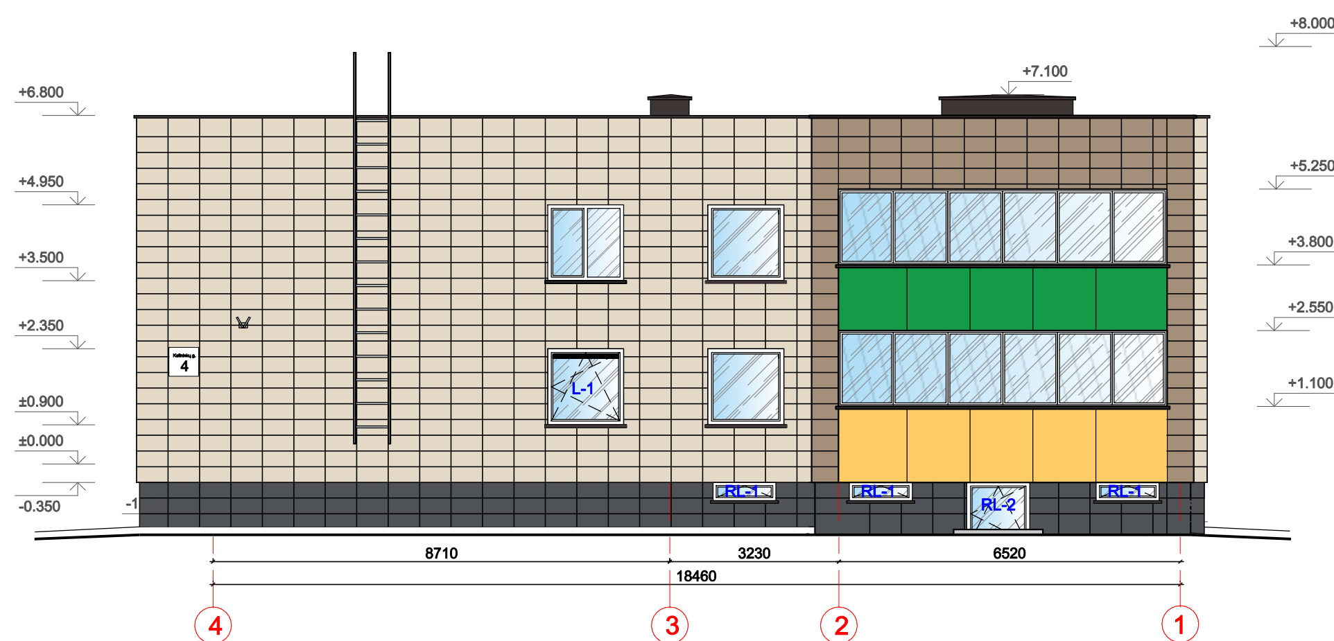
FASADAS TARP AŠIŲ "4-1" M 1:100
