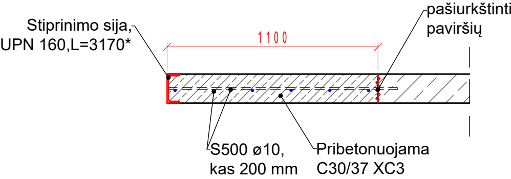
PJŪVIS B-B M 1:50
