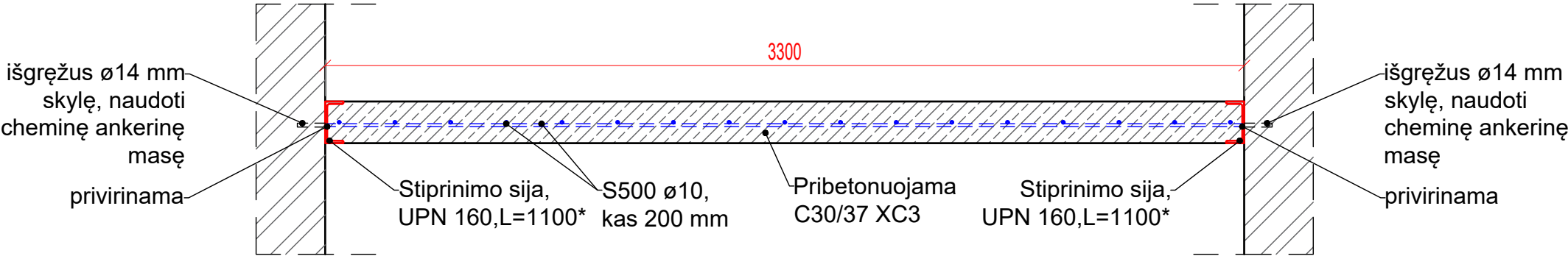
PJŪVIS A-A M 1:50
