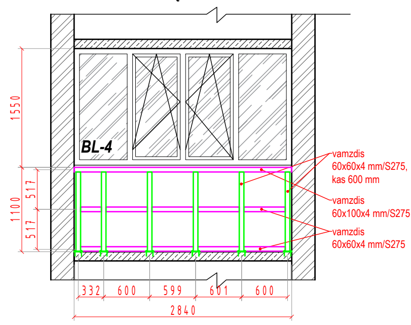
LODŽIJŲ ATITVARO BL-4 ĮRENGIMAS TARP AŠIŲ "D-C" M 1:50
