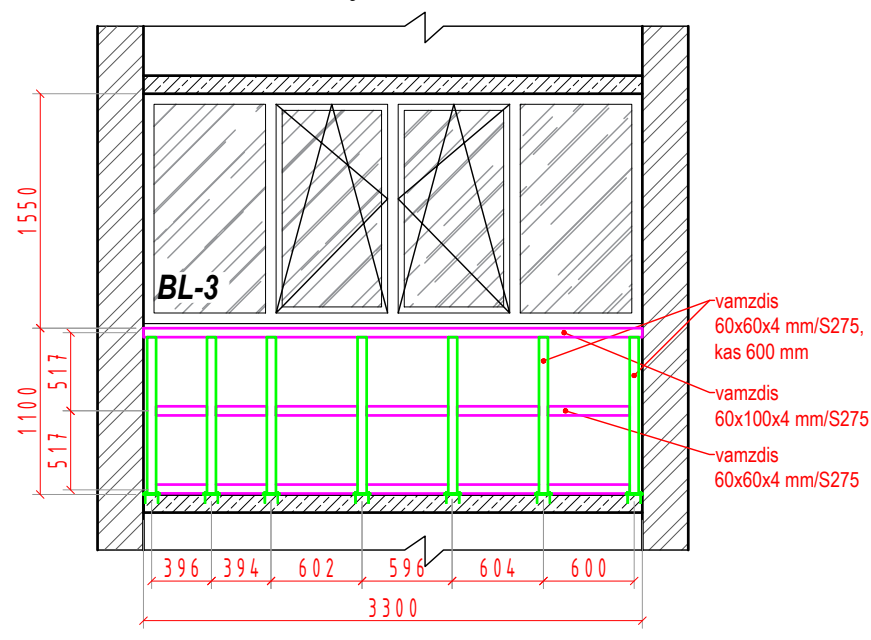
LODŽIJŲ ATITVARO BL-3 ĮRENGIMAS TARP AŠIŲ "4-3" M 1:50
