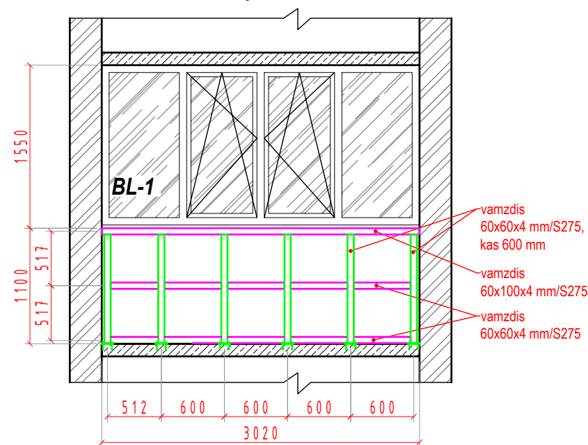
LODŽIJŲ ATITVARO BL-1 ĮRENGIMAS TARP AŠIŲ "5-6" M 1:50
