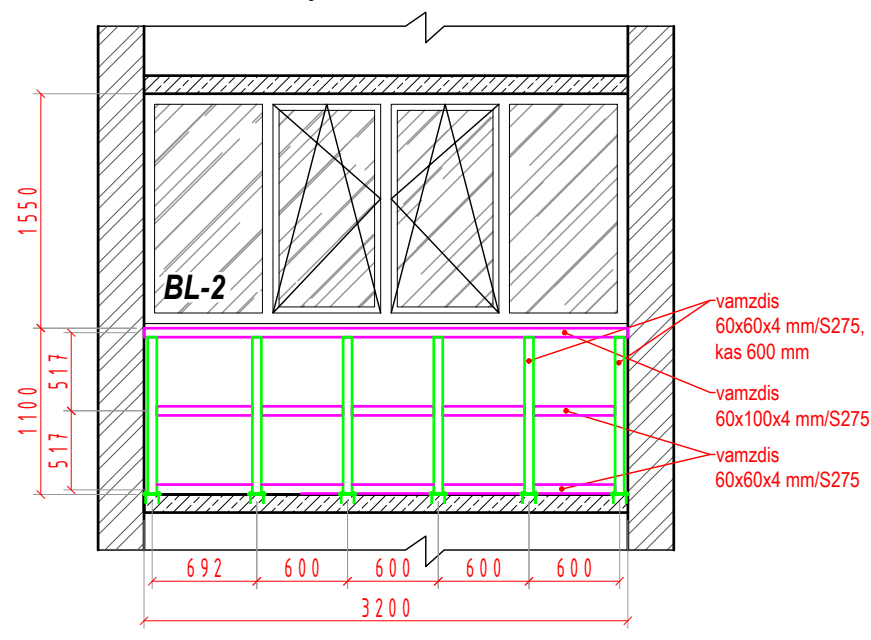
LODŽIJŲ ATITVARO BL-2 ĮRENGIMAS TARP AŠIŲ "D-E", "5-4" M 1:50
