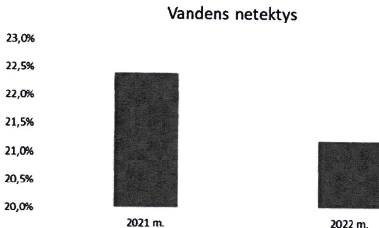
4 pav. 2021 m. ir 2022 m. vandens netekčių palyginimas
